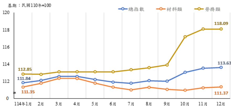
臺中市 114 年營造工程物價指數走勢圖
